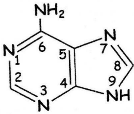
Adénine
